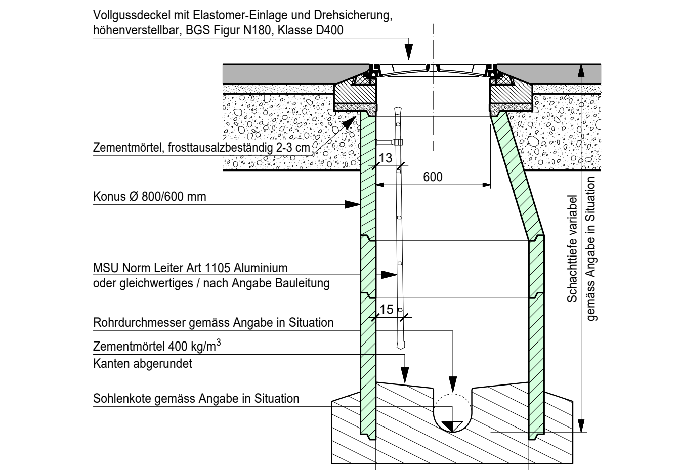
Kontroll-/Einstiegschachtschacht Ø 1000/600mm, 1:20
