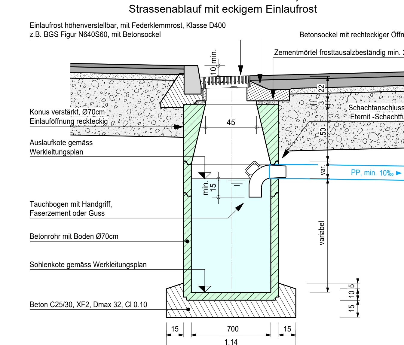
Systemaufbau 1:20
