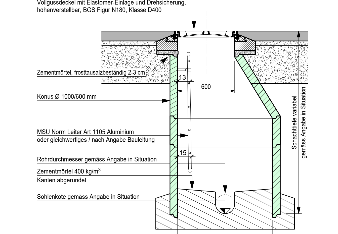
Strassenablauf Ø700mm, 1:20
