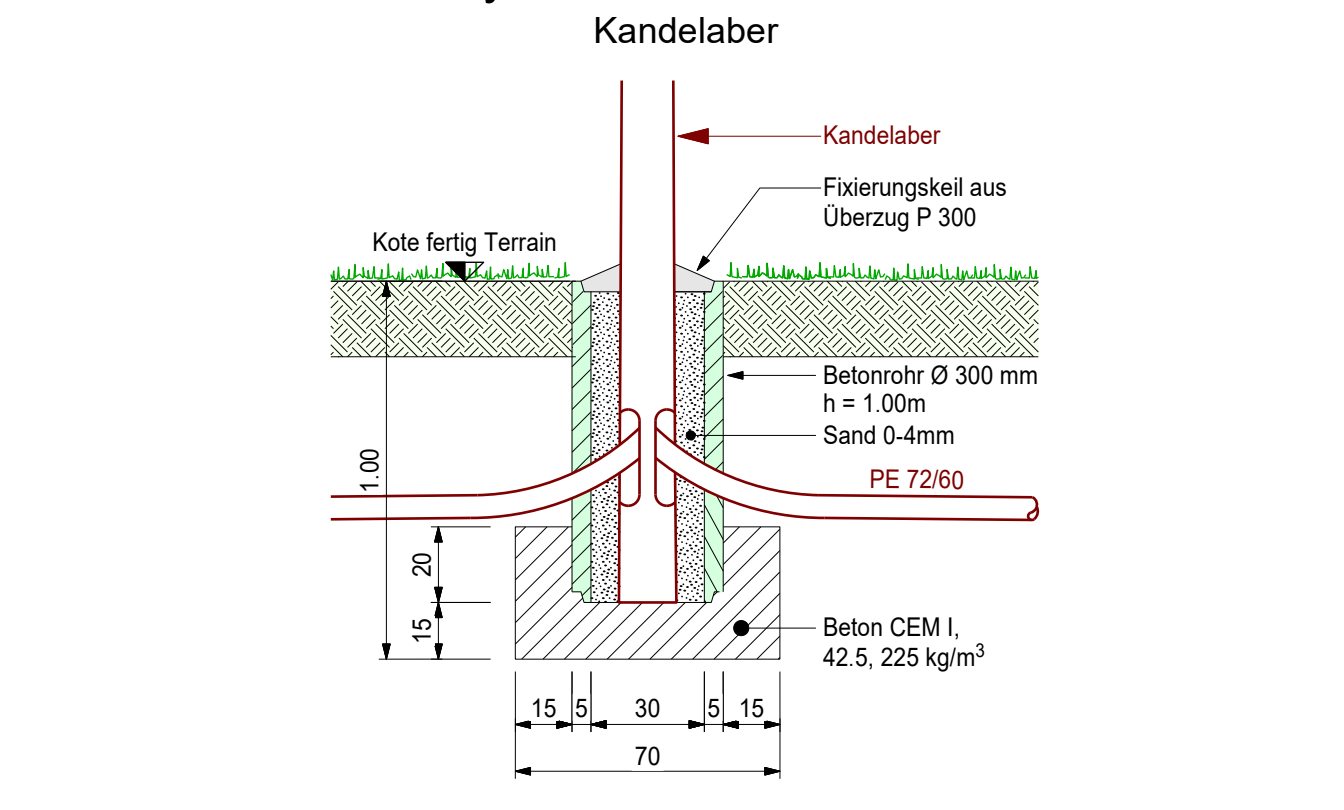
Systemaufbau 1:20
